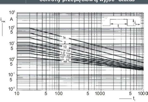
Rys. 12 Maks. liczba impulsów prądowych w zależności od czasu ich trwania dla ochrony przepięciowej wyjść "Status"
