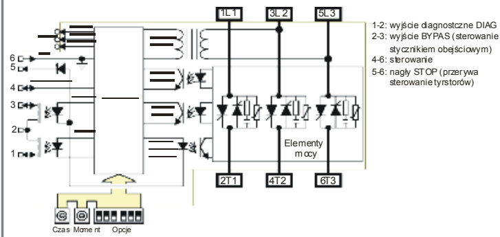
Rys. 1 Schemat wewnętrzny
