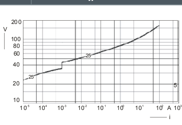
Rys. 11 Charakterystyka ochrony przepięciowej wyjścia "Status"
