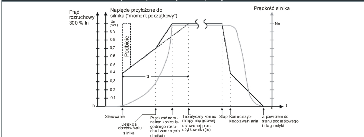
Rys. 3 Opis różnych faz pracy silnika
