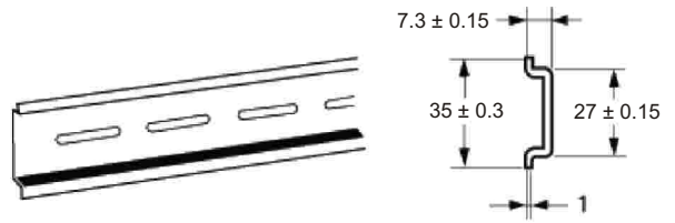
Wymiary szyny DIN
