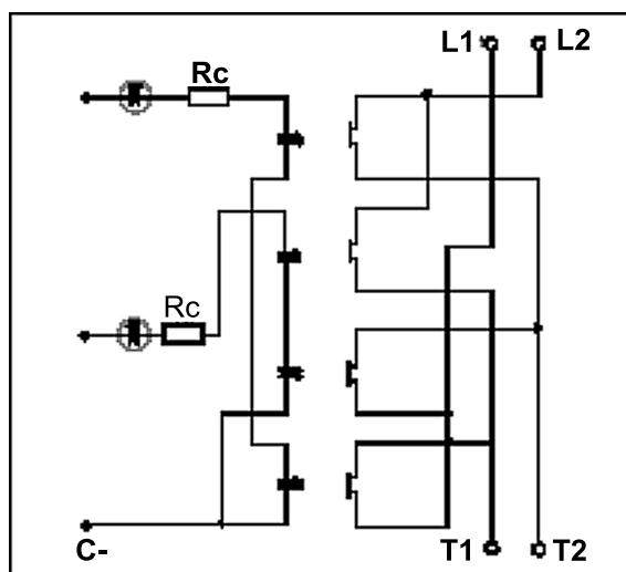
Schemat wewnętrzny XKRD 30506
