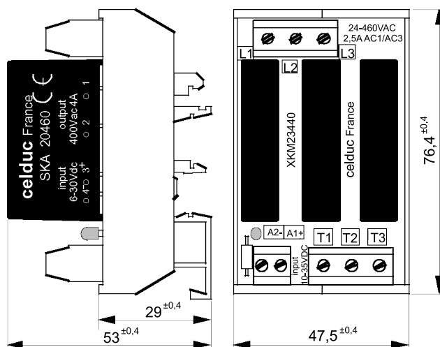
XKM23440: wymiary (mm)
