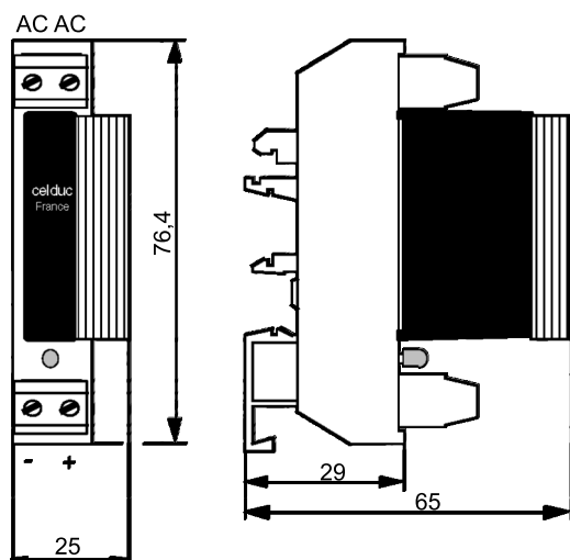
XKM22440: wymiary (mm)
