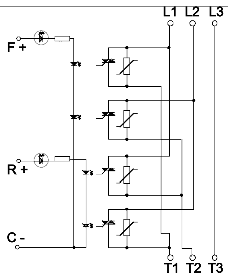
XKRD 30506: typowa aplikacja
