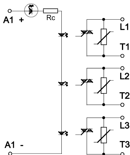
Schemat wewnętrzny XKM23440
