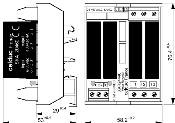
XKR24440: wymiary (mm)
