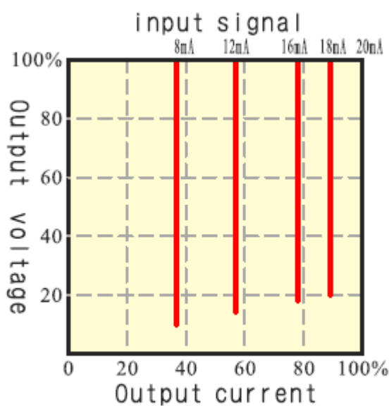
Stały prąd wyjściowy
