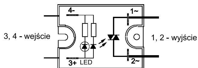
Schemat wewnętrzny:
