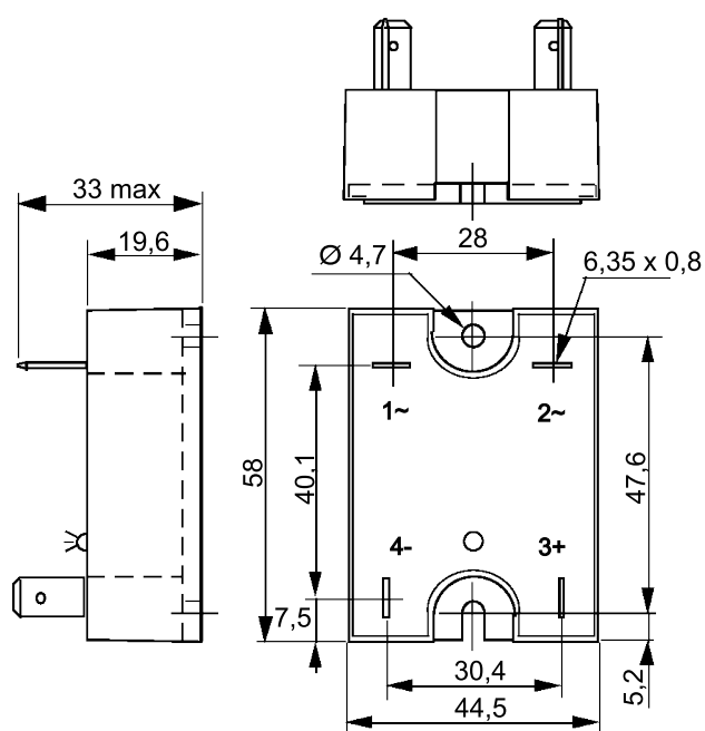
Wymiary (mm):
